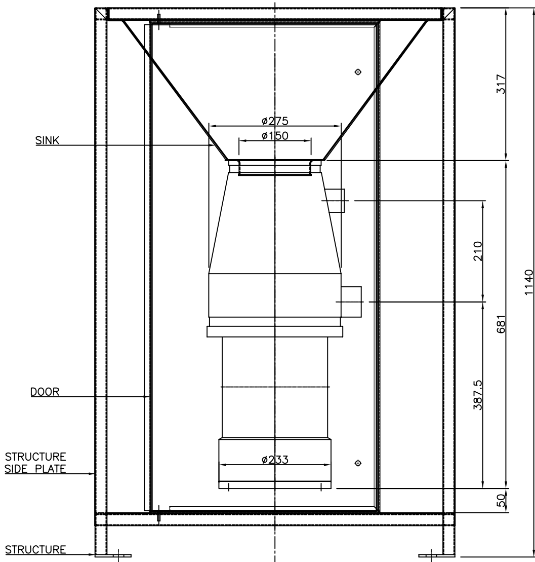
ELEVATION
